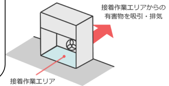
囲い式局所排気装置
